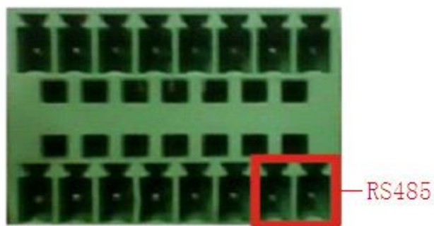
Interfejs 485 dla rejestratora z 8 wejściami alarmowymi
