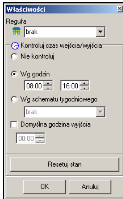
Rys. 37. Okno WŁAŚCIWOŚCI.
